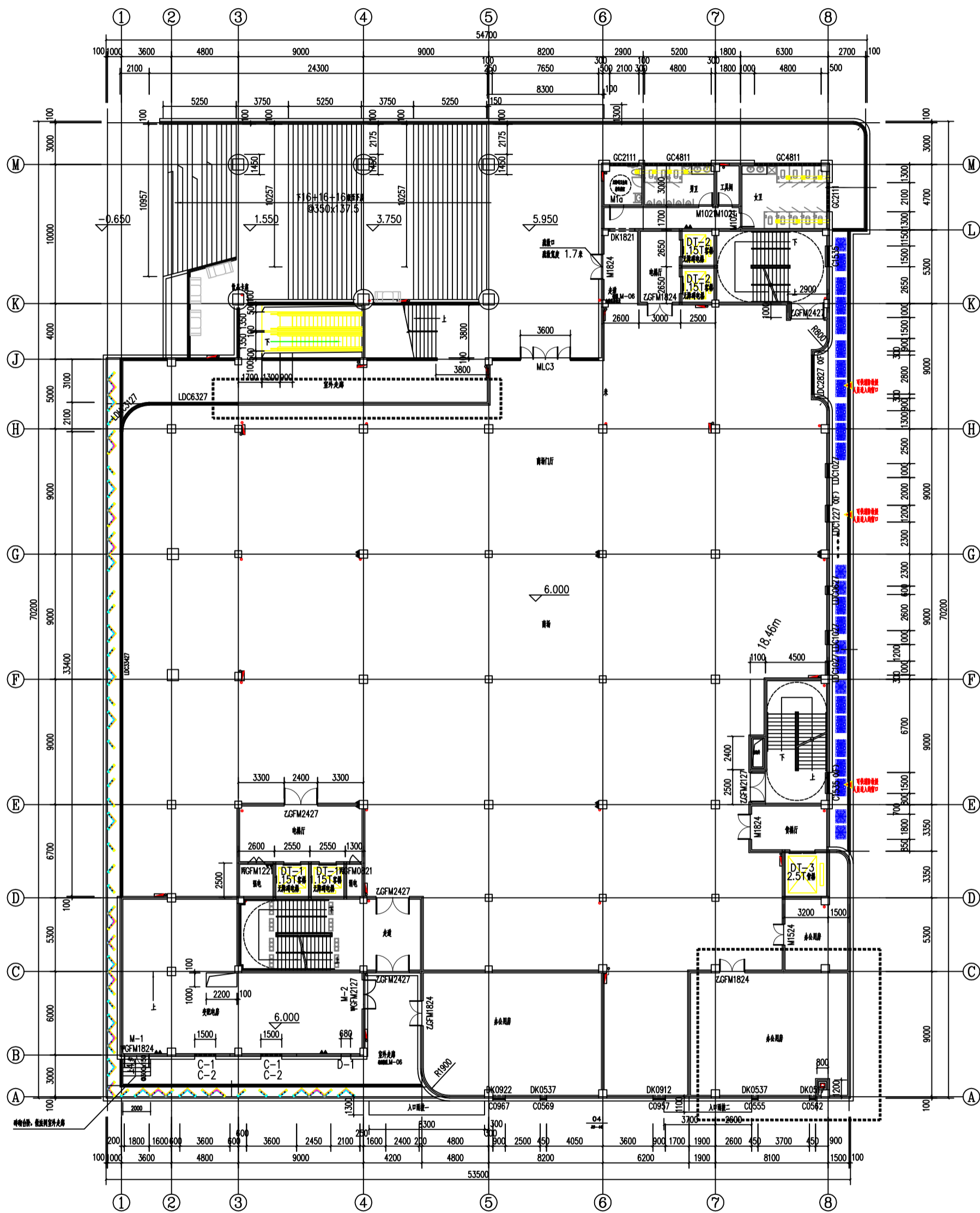
二层平面图 1:150
