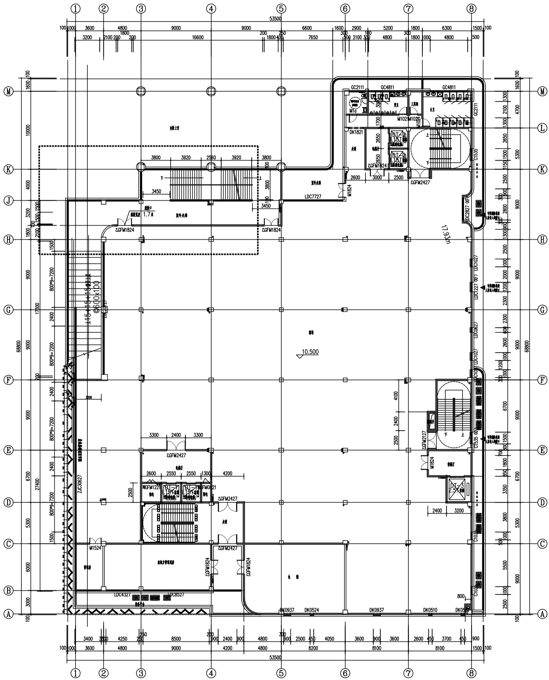
三层平面图 1:150
