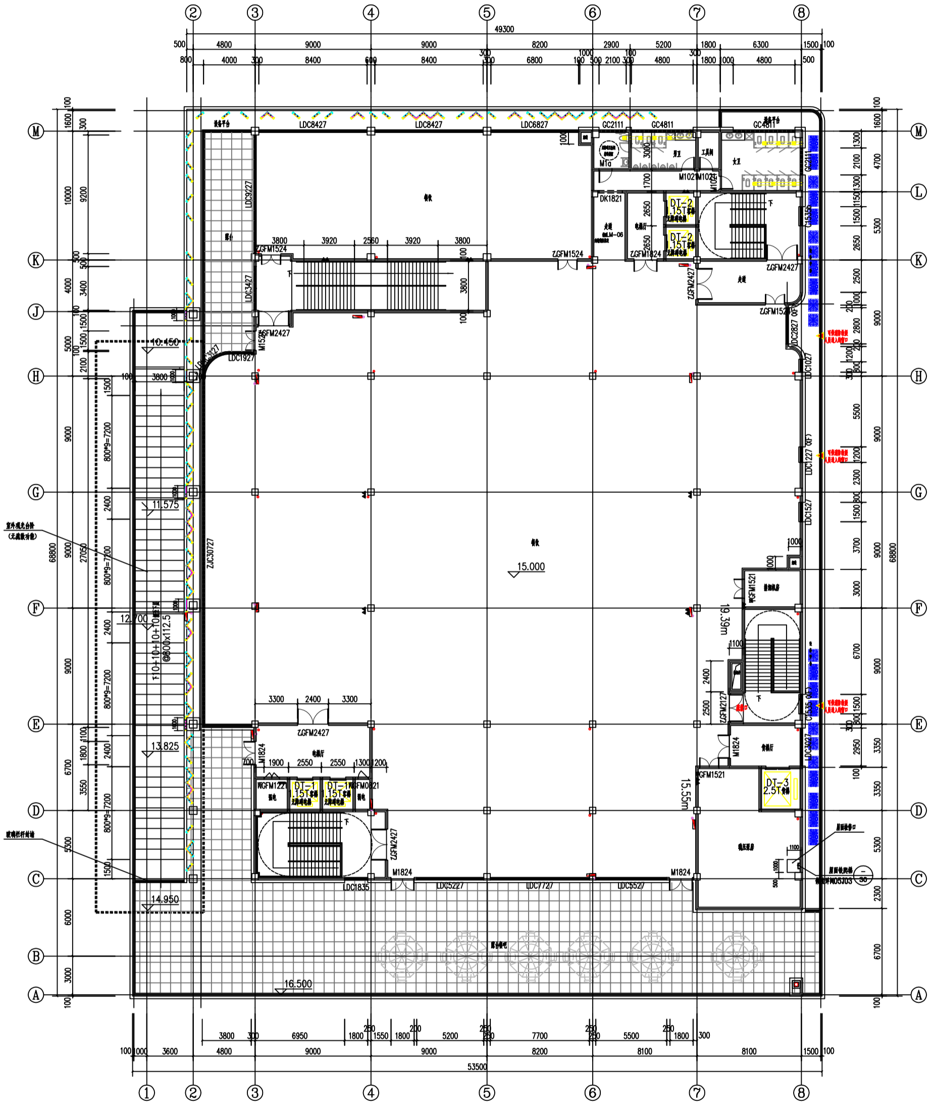
四层平面图 1:150
