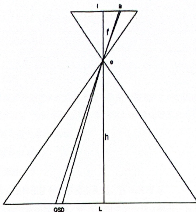
图2 航高与地面采样距离关系
